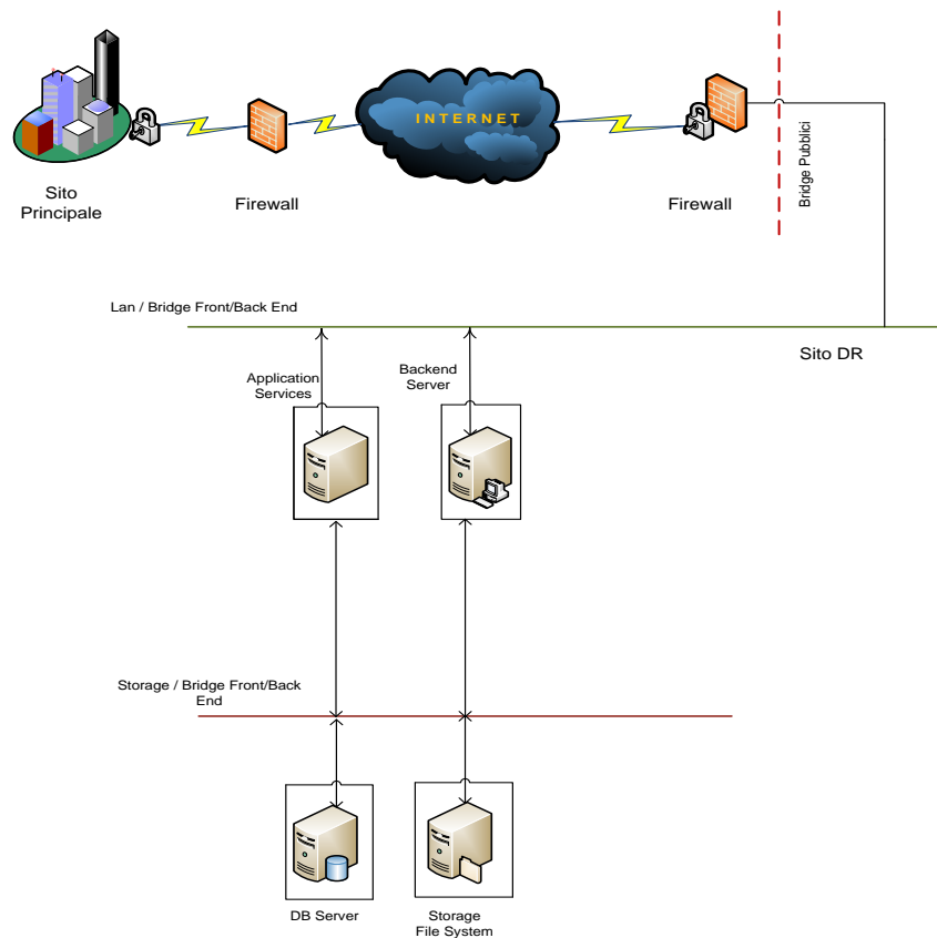
Figura 14 Macro architettura di collegamento del sito di DR
